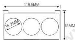
ES1117-3YNT(ES1117C-3YNT) ES1179W-3YNT ES1179H-3YNT ES1179HW-3YNT
