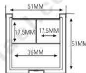
ES1087-2FS(ES1087A-3) ES1087L-2FS(ES1087LA-3) ES1087S-2FS
