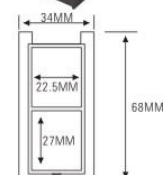
ES1153-2F SIZE: L34×W68×H18.3mm
