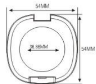
ES1097 SIZE: L54×W54×H20.8mm
