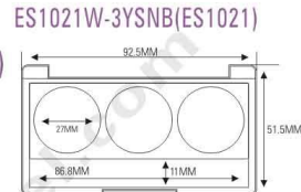
ES1021W-3YSNB(ES1021) ES1021W-2Y36(ES1021-2Y36) ES1021W-2F(ES1021-2F) SIZE: L92.5×W51.5×H11.5mm
