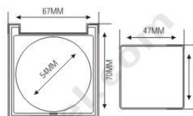
ES1085B-1R SIZE: L67×W70×H23mm
