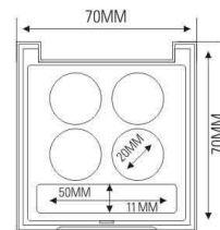
ES1086-4YS(ES1086C-4R) SIZE: L70×W70×H18mm
